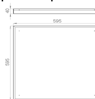
Габаритный чертеж светильника
